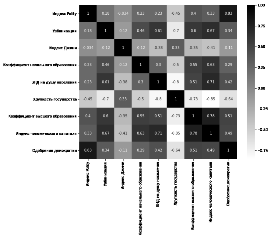
Рис. 2. Матрица корреляций
