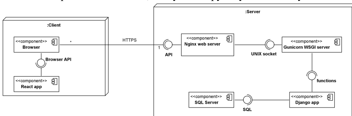
Рис. 6. Физическая структура системы
