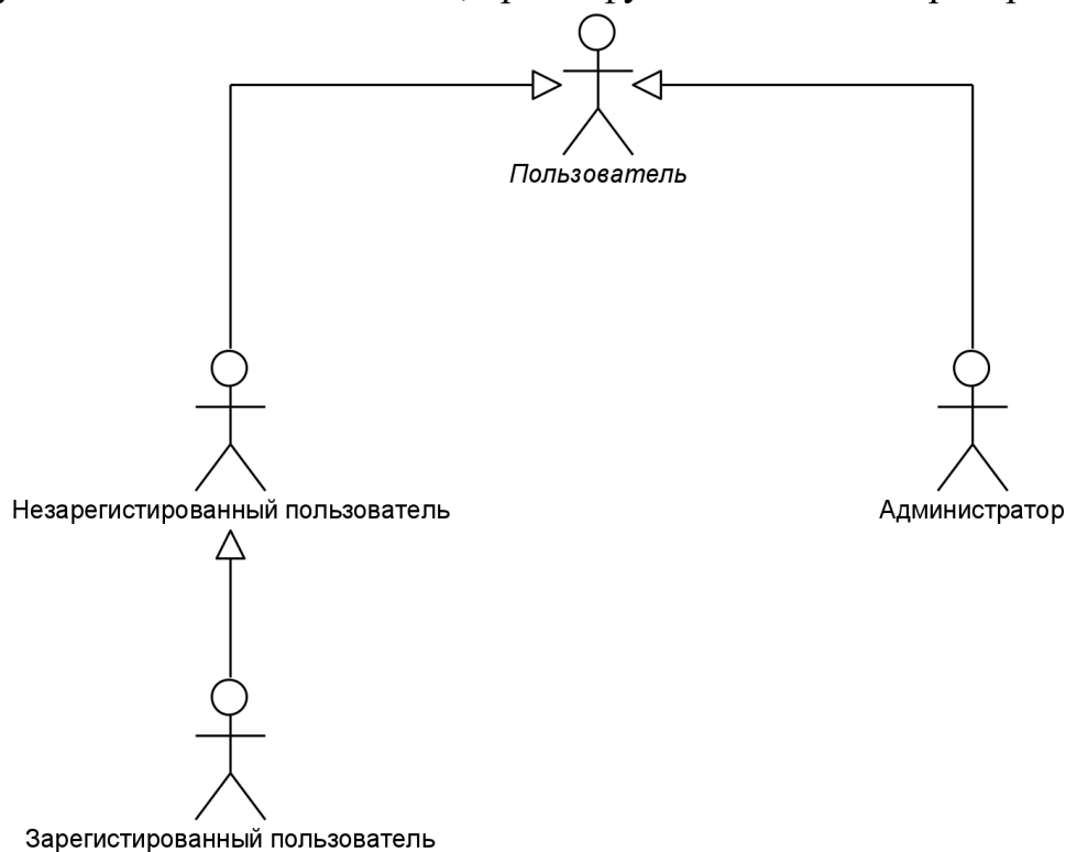
Рис. 1. Иерархия акторов
