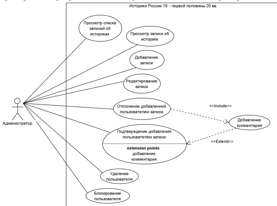
Рис. 5. Возможности администратора
