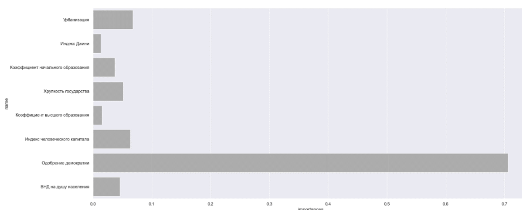
Рис. 4. Важность признаков
